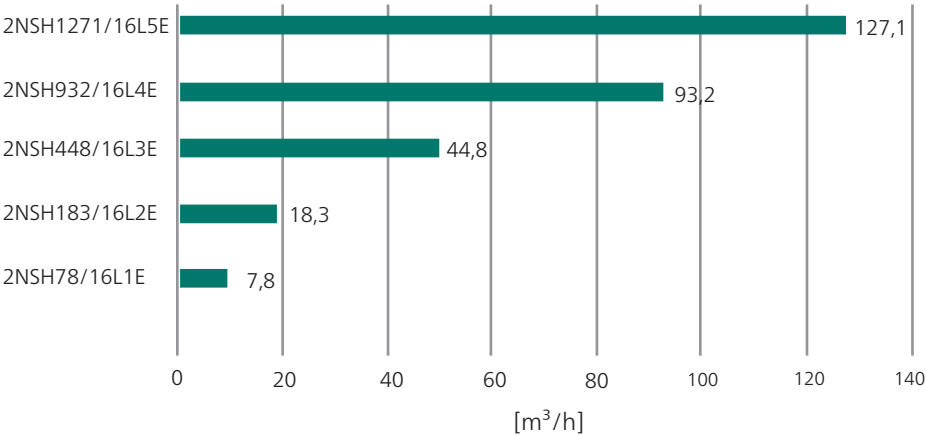
Flujo máximo de cada serie de bombas
