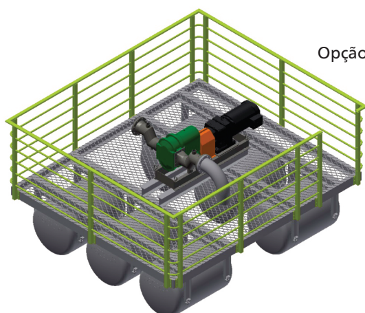
Projeto TORNADO® flutuante
